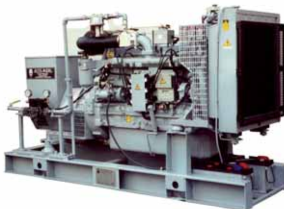
MOD. GF135C6ST15/3 GRUPPO ELETTROGENO DA 100 KVA CON MOTORE CICLO OTTO A GAS
